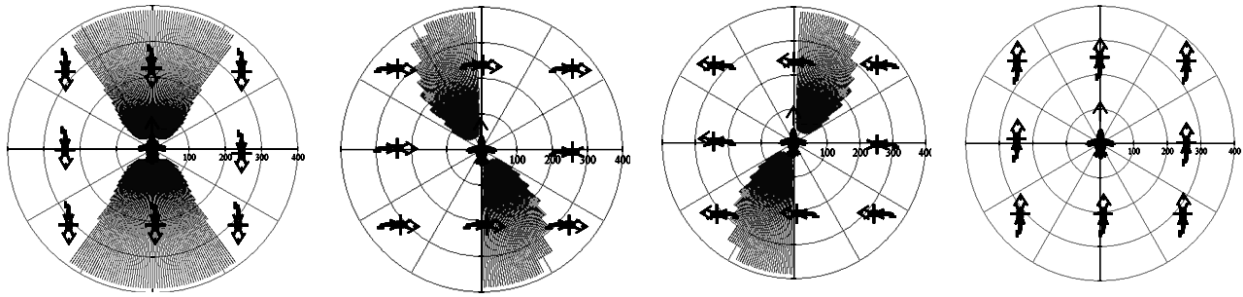
Рис. 5. Зони виявлення малошвидкісних цілей типу вертоліт ( \sigma_c=2 \text{ м}^2 ) літаком ДРЛВіУ типу Е-3А при H_{ц}=9 \text{ км} , V_{ц}=200 \text{ м/с} , \beta_{ц}=0^\circ , H_{ц}=100 \text{ м} , V_{ц}=50 \text{ м/с} та різних ракурсах цілі
