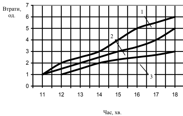
Рис. 4. Залежність втрат ББМ від складу комплексу озброєння: 1 – 105-мм гармата; 2 – 30-мм МАГ (ОФС); 3 – 40-мм МАГ (ОФС з дистанційним підризником).
