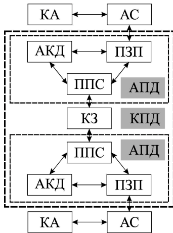
Рис. 5. Типова схема елемента підсистеми зв'язку
