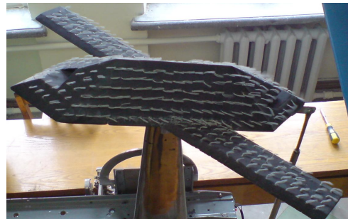
Рис. 11. Фотографія спектру обтікання моделі з крилом прямої стріловидності при \alpha = 10^\circ
