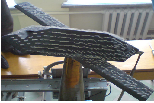
Рис. 13. Фотографія спектру обтікання моделі з крилом прямої стрілоvidності при \alpha = 14^\circ
