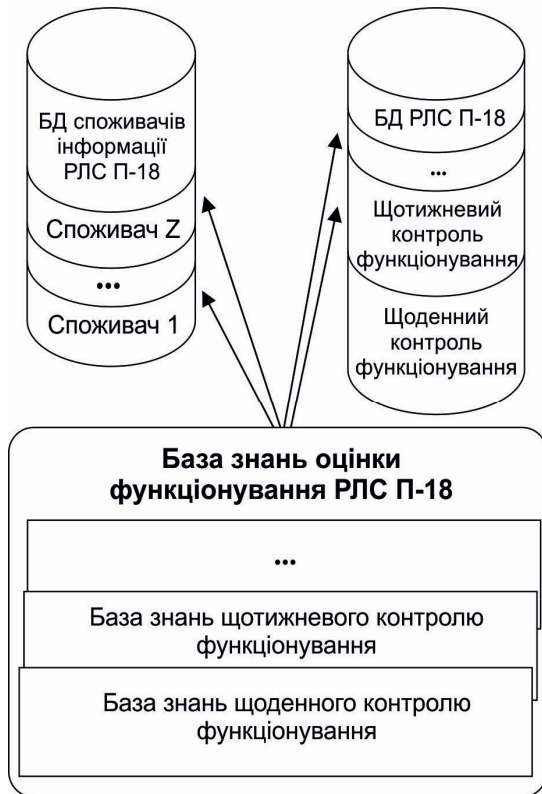
Рис. 2. Логічна структура оцінки стану РЛС П-18
