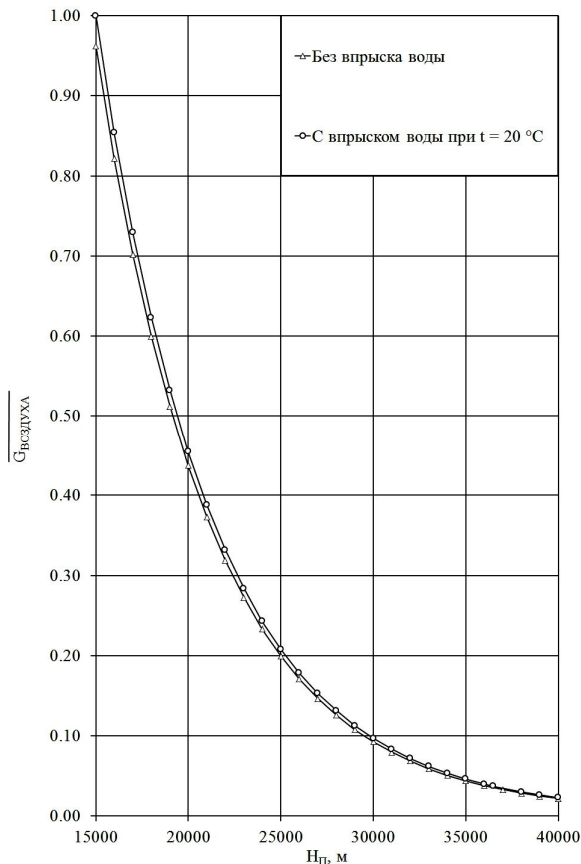
Рис. 10. Влияние впрыска воды на расходную характеристику воздухозаборника при скорости полета M_{\text{П}} = 5
