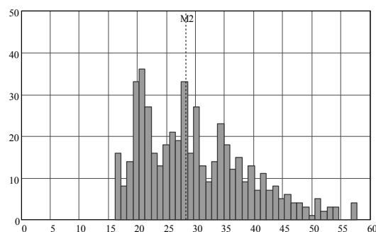
Рис. 3. Распределение кодовых слов LFSR ПСК при n = 5
