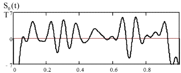
Рис. 5. Комплексная огибающая сигнала S_0(t) при n=16
