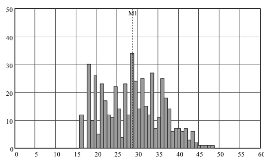
Рис. 2. Распределение кодовых слов ЛКГ ПСК при n = 5
