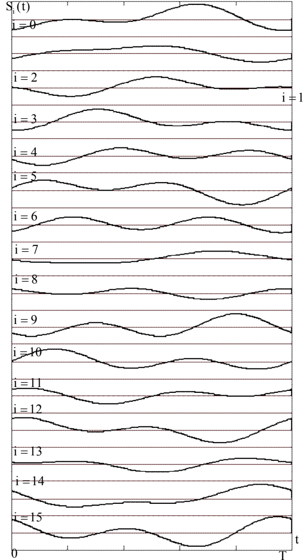
Рис. 4. Комплексные огибающие сигналов кодовой книги ПСК ЛКГ при n=4 .
