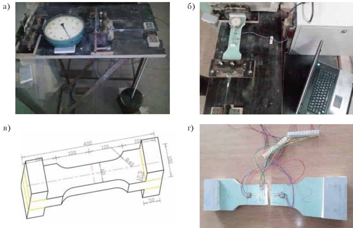
Рисунок 2. Испытания на осевое растяжение: а) тарировка опытной установки; б) замеры деформаций при нагружении; в) размеры опытных образцов; г) характер разрушения образцов.
