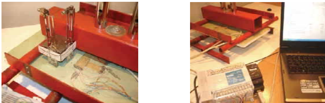
Рисунок 3. Контроль деформаций с помощью тензорезисторов и тензометров Гугенбергера.
