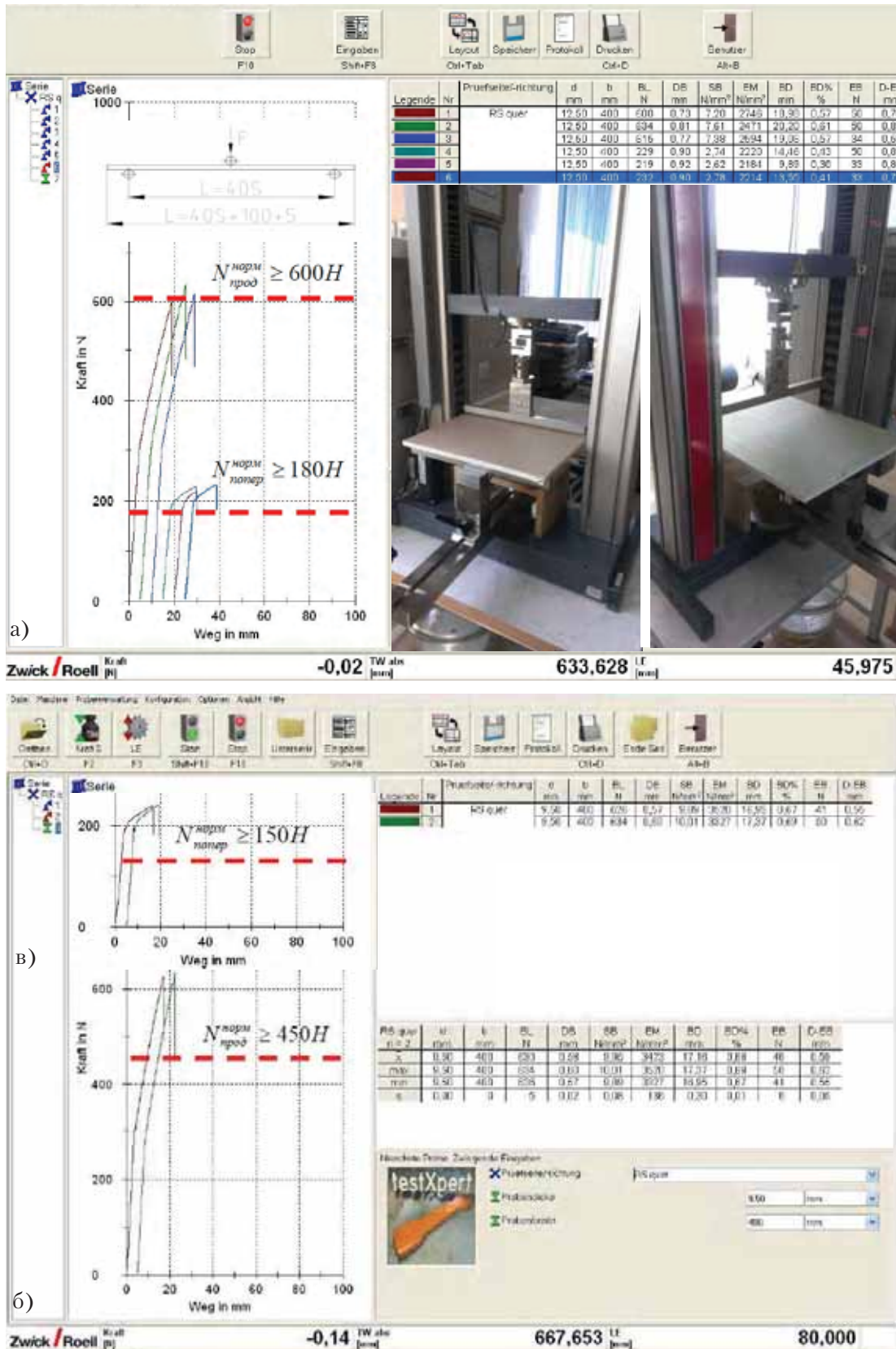
Рисунок 1. Результаты испытания по ГОСТ 6266-97 при переменном пролете продольных и поперечных образцов из: а) ГКП 12,5 мм, б), в) ГКП 9,5 мм на сертифицированном оборудовании Zwick Roell.
