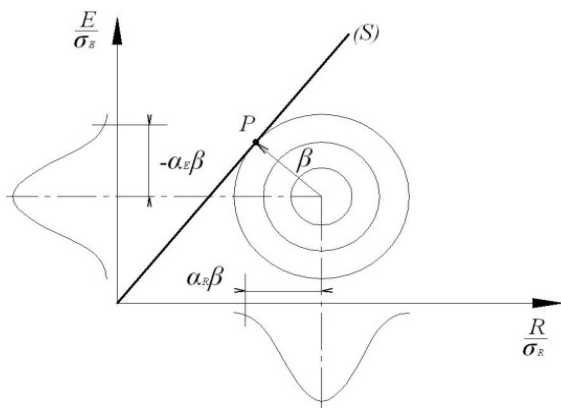
Рисунок 1. Характеристика безопасности в пространстве случайных переменных E, R : (S) – граница безопасной зоны; P – проектная точка.
