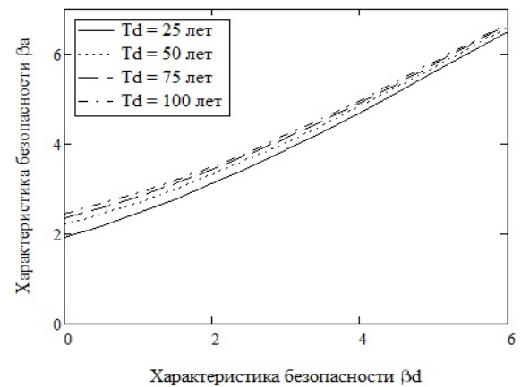
Рисунок 2. Зависимость характеристики безопасности \beta_1 для базового периода повторяемости в один год от проектной характеристики безопасности \beta_d при различных значениях проектного срока службы T_d .
