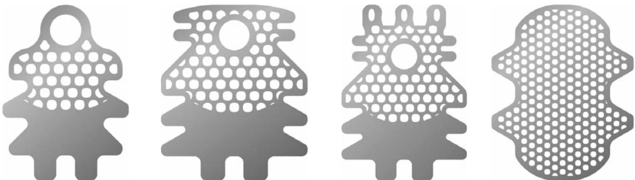
Рис. 4. Титановые мембраны СТИ-мет.
