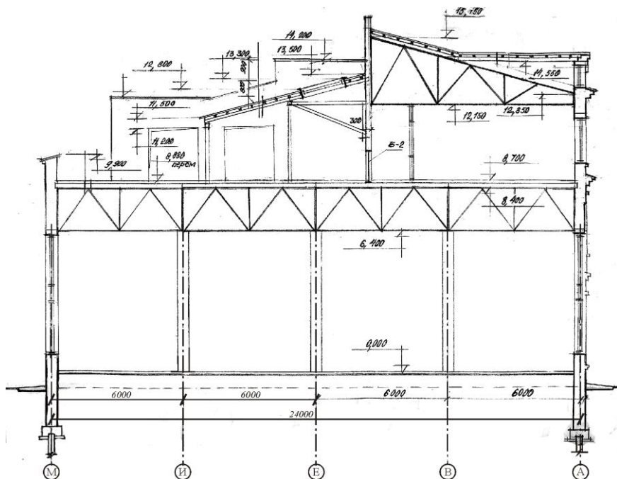
Рис. 1. Поперечный разрез рассматриваемого здания
