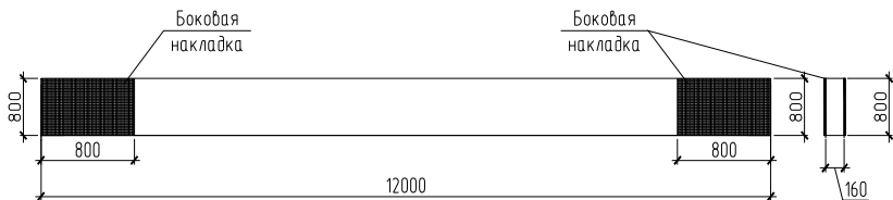
Рис. 5. Расчетная схема балки с боковыми накладками из сеток
