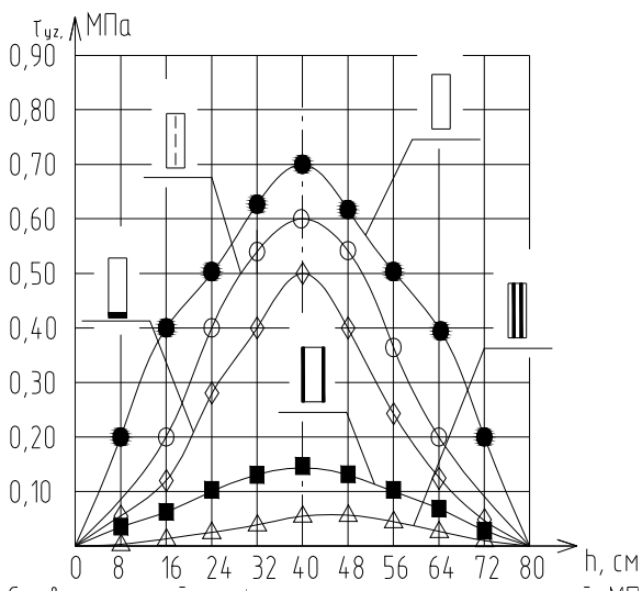
Рис. 6. Сравнительные графики (эпюры) касательных напряжений разных схем усиления балок
