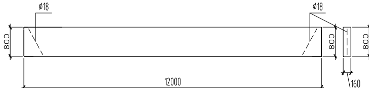
Рис. 2. Расчетная схема балки с наклонно-вклеенными стержнями
