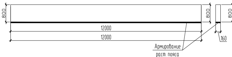
Рис. 4. Расчетная схема балки с послойным армированием сетками растянутого пояса
