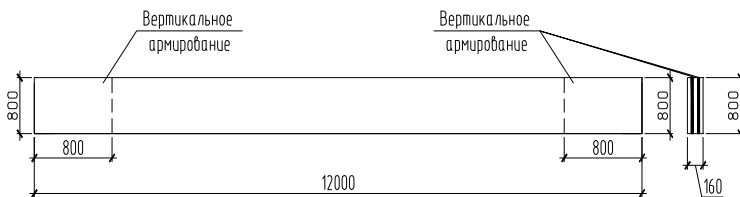
Рис. 3. Расчетная схема балки с армированием сетками в опорной части
