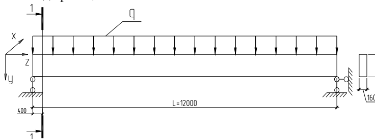
Рис. 1. Расчетная схема балок
