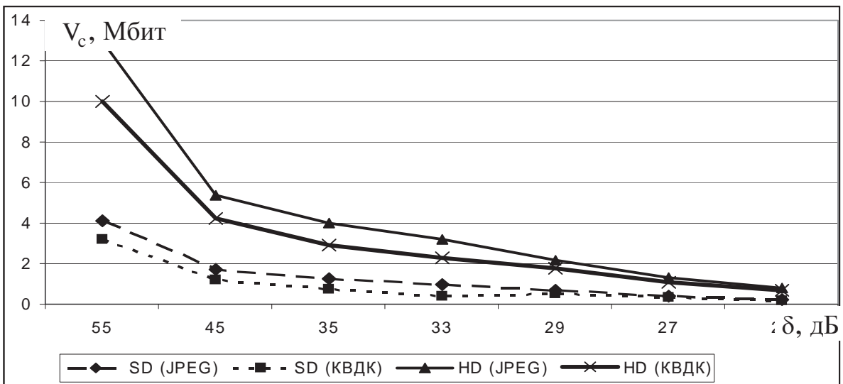
Рис. 2. Графики зависимости битовой скорости кадра от ПОСШ для разного пространственного разрешения
