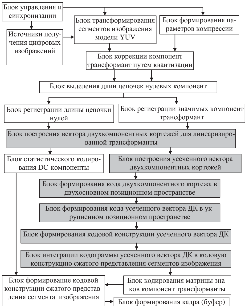
Рис. 1. Схема интеграции кодового представления усеченного вектора двухкомпонентных кортежей в технологию сжатия на платформе JPEG
