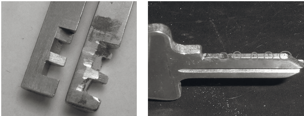
Рис. 19. Візуалізація трас від кодових елементів при виконанні імпресії (а – для дискового механізму; б – для штифтового механізму)
