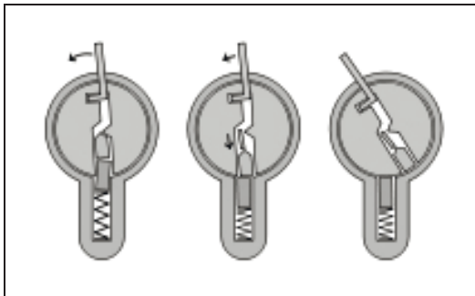
Рис. 21. Відкриття замка за допомогою відмички (а – алгоритм деблокування циліндру з вертикальним розташуванням замкової шпарини; б – типові відмички та натяжки для штифтового механізму)
