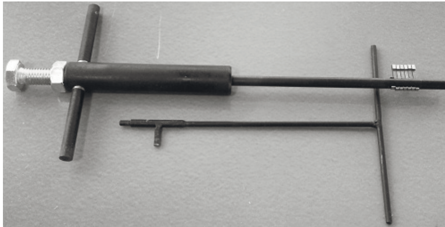
Рис. 25. Набір інструментів для самоімпресії (зверху – зчитувач кодівих рівнів; знизу – натяг)
