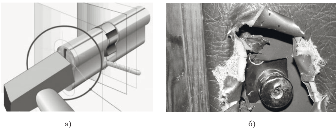
Рис. 16. Вилучення механізму секретності (а – вибиття циліндру всередину приміщення; б – відривання від корпусу замка)
