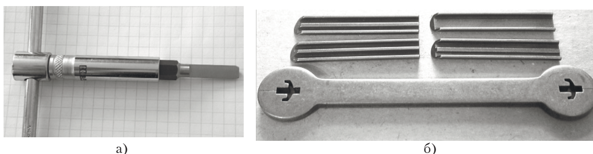
Рис. 15. Інструменти для зрізання стопорних елементів циліндра
