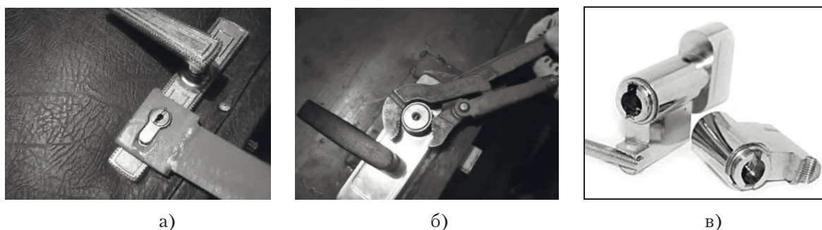
Рис. 14. Злам корпусу механізму секретності
