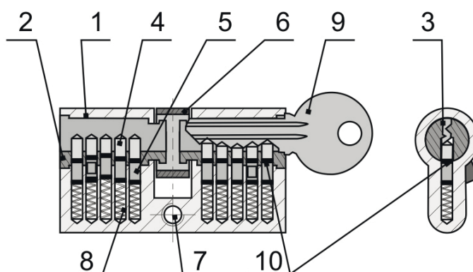
Рис. 9. Механізм секретності циліндрового замка
