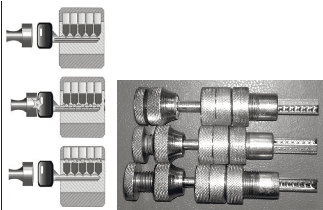
Рис. 17. Принцип та обладнання для реалізації бампінгу
