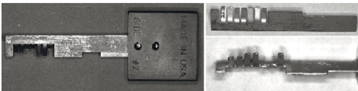
Рис. 20. Обладнання для отримання коду ключа методом самоімпресії (а, б – для штифтового циліндру з вертикальним та горизонтальним розташуванням замкової шпарини; в, г – для дискового механізму фінського типу)
