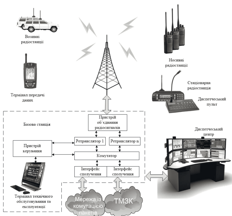
Рис. 2. Однозонова транкінгова система
