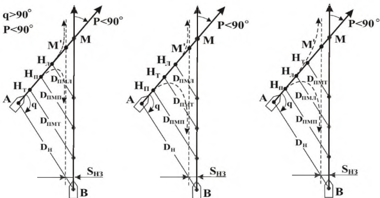
Рис 2. Расчетная схема для оптимизации выбора маневра последнего момента
