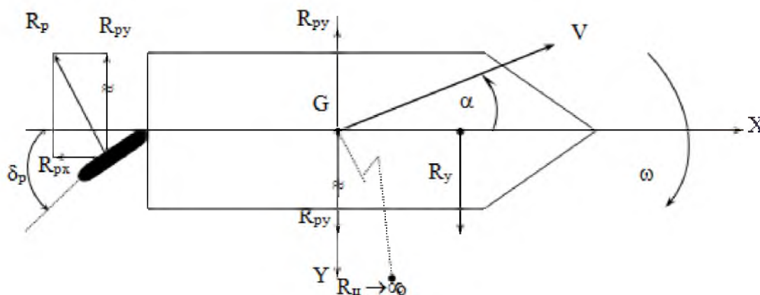
Рис. 1 Силы, действующие на судно с переложенным рулем в начальной стадии поворота судна.
