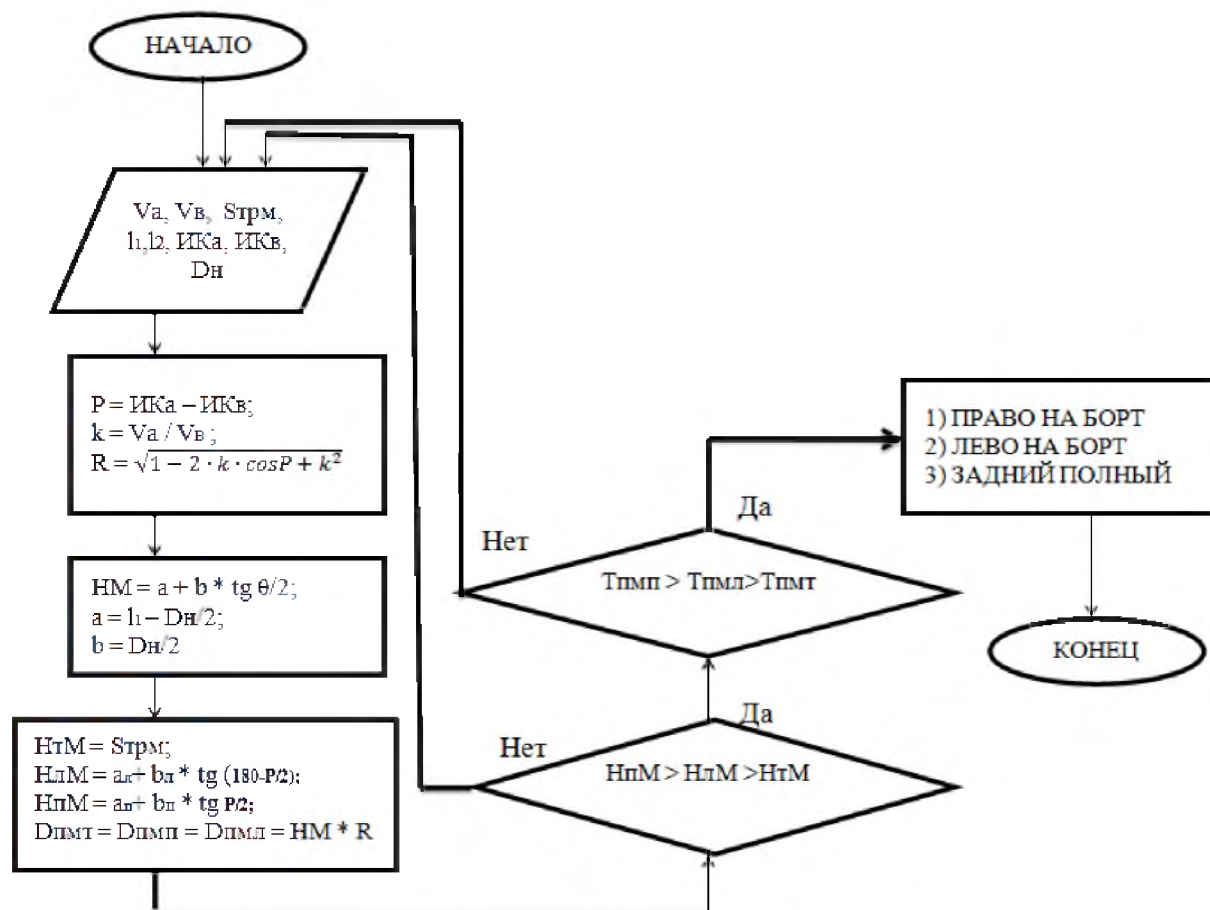
Рис. 3 Блок-схема алгоритма расчета вида маневра
