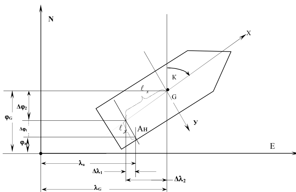
Рис. 1 Приведение observations к центру тяжести судна
