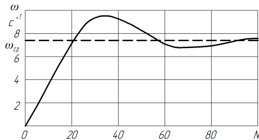
Рис. 3. Графік зміни миттєвої швидкості обертання ротора на частоті швидких переміщень
