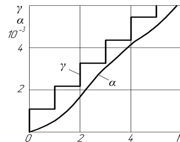
Рис. 4. Графіки кутових характеристик при неграничному пуску
