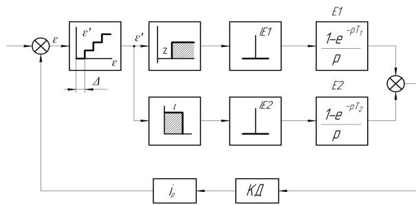
Рис. 1. Структурна схема двохшвидкісного крокового електроприводу
