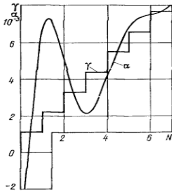
Рис. 5. Графіки кутових характеристик у режимі перемикання \gamma_{max} = f(N) та \alpha_{max} = f(N)
