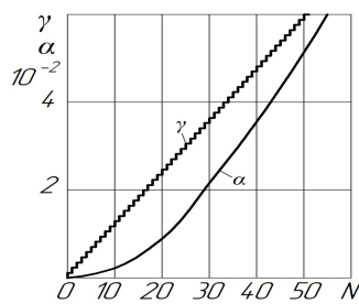
Рис. 2. Графіки кутових характеристик при пуску двигуна на частоті швидких переміщень
