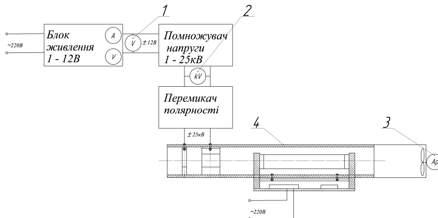
Рис. 1. Схема експериментальної установки для визначення параметрів іонновітрового бактерицидно-озонатора: 1 – вольтметр; 2 – кіловольтметр; 3 – ареометр АСО-3; 4 – зnezаражувач-озонатор
