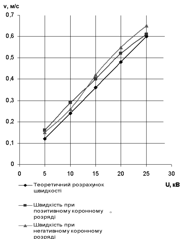
Рис. 2. Залежність швидкості вітру від напруги на електродах іонновітрового бактерицидного знезаражувача-озонатора V_e = f(U) .
