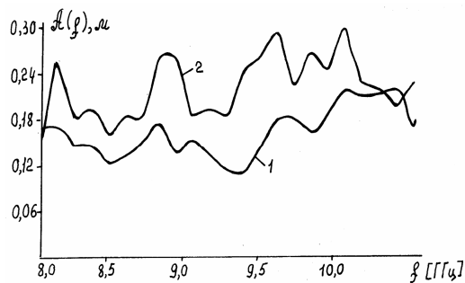
Рис. 5. Частотная зависимость амплитуды для РПМ второго типа
