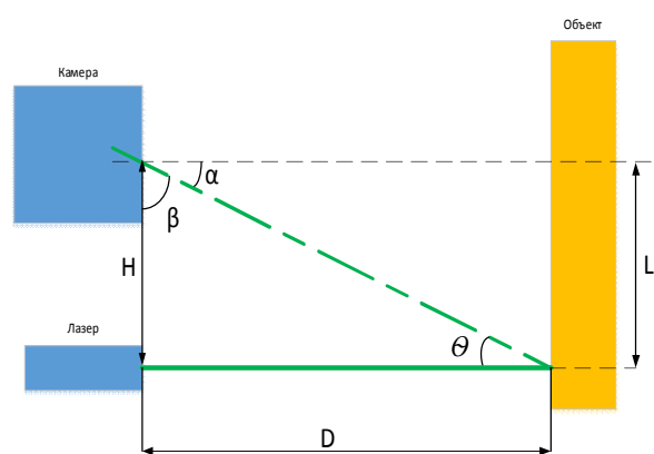
Рис. 1. Лазерная триангуляция
