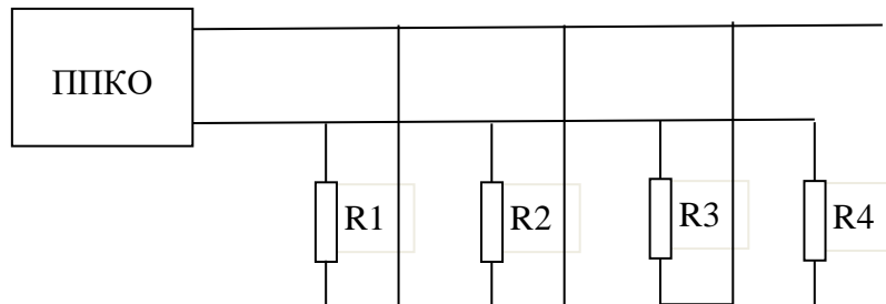
Рис. 5 Еквівалентна електрична схема шлейфної структури з резисторами
