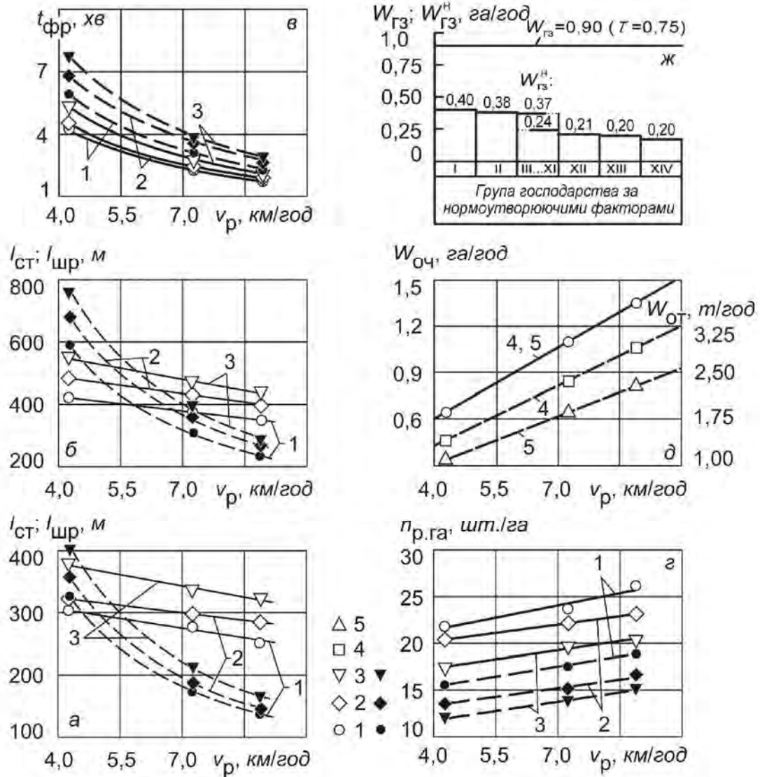
Рис. 2 – Вплив швидкості руху v_p прес-підбирачів на зміну: а) довжини піднятої з поля стрічки трести l_{\text{СТ}} (суцільної лінії) для формування одного рулону і довжини шару стебел в рулоні l_{\text{ШР}} (пунктирні лінії) при використанні прес-підбирача ПР-1,2Л; б) те ж прес-підбирача ППР-110; в) тривалості формування рулону t_{\text{ФР}} і з) їх кількості на 1 га зібраної площі n_{\text{р.га}} при використанні прес-підбирача ПР-1,2Л (суцільні лінії) і ППР-110 (пунктирні) за установки регулятора щільності рулонів в положення мінімальне (1), основне (2) і максимальне (3); д) продуктивності агрегату за годину основного часу в тоннах піднятої трести W_{\text{ОТ}} (т/год) і зібраної площі W_{\text{ОЧ}} (га/год) у складі з прес-підбирачем ПР-1,2Л (4) і ППР-110 (5); ж) прогнозована продуктивність агрегатів з прес-підбирачами за годину змінного часу W_{\text{ГЗ}} (га/год) і годинна норма продуктивності W_{\text{ГЗ}}^H з урахуванням групи господарства за нормоутворюючими факторами
