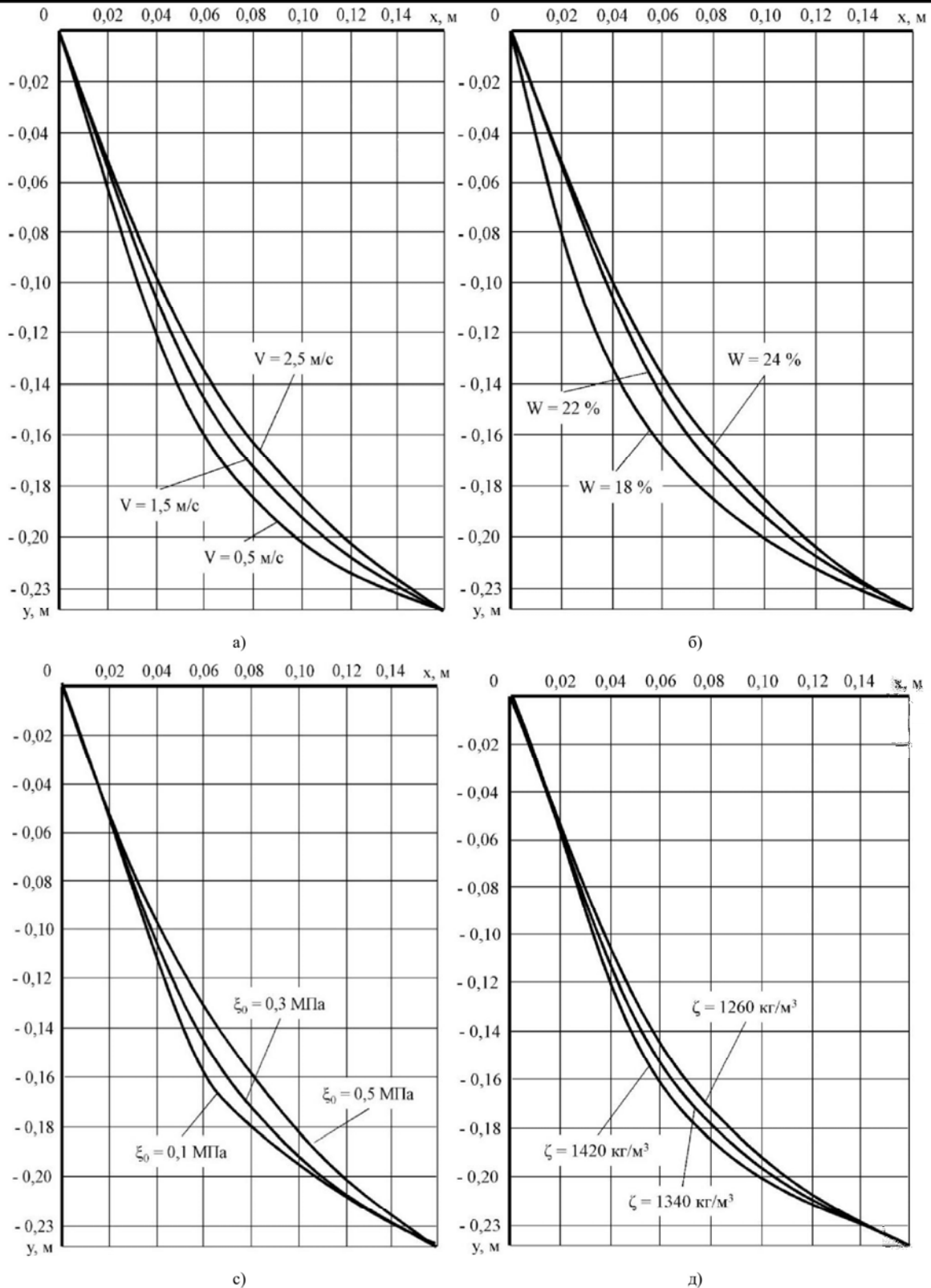
Рис.1 – Геометрична форма поверхні лани культиватора в залежності від: а) швидкості її переміщення; б) вологості ґрунту; в) коефіцієнту бокового тиску; д) щільності ґрунту
