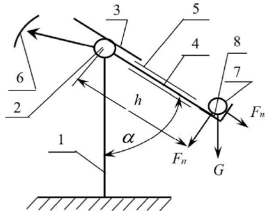
Рис. 1 – Калібрувальна схема вимірювача маси потоку дисперсних матеріалів: 1 – опора; 2 – позовжня балка; 3 – компенсатор динамічних зусиль; 4 – тензовимірювальна площина; 5 – тензодатчик; 6 – механізм зміни кута нахилу тензовимірювальної площини; 7 – гирі; 8 – фіксована пластина для гир
