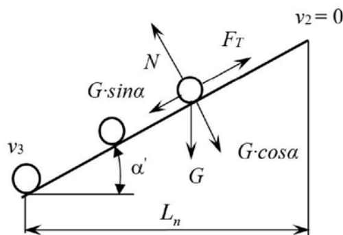
Рис. 5 – Схема дії сил на елементарну частинку сипкого матеріалу при русі її по вимірювальній площині
