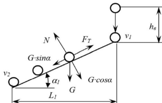
Рис. 4 – Схема дії сил на елементарну частинку комбікорму при її русові на компенсаторі динамічних зусиль: G – сила маси, Н; N – сила нормальної реакції, Н; F_T – сила тертя, Н
