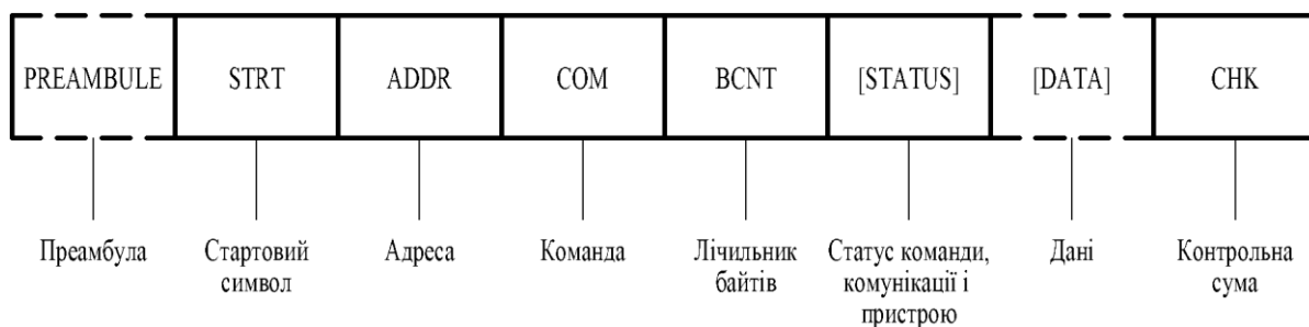
Рис. 1. Структура HART-повідомлення
