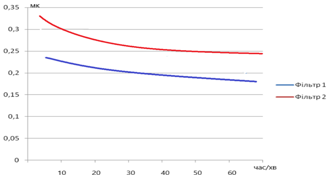
Рис. 3. Показання датчику забруднення повітря (PMS50-03): фільтр 1 – запропонований нами фільтр CH-8450D ; фільтр 2 – серійний фільтр
