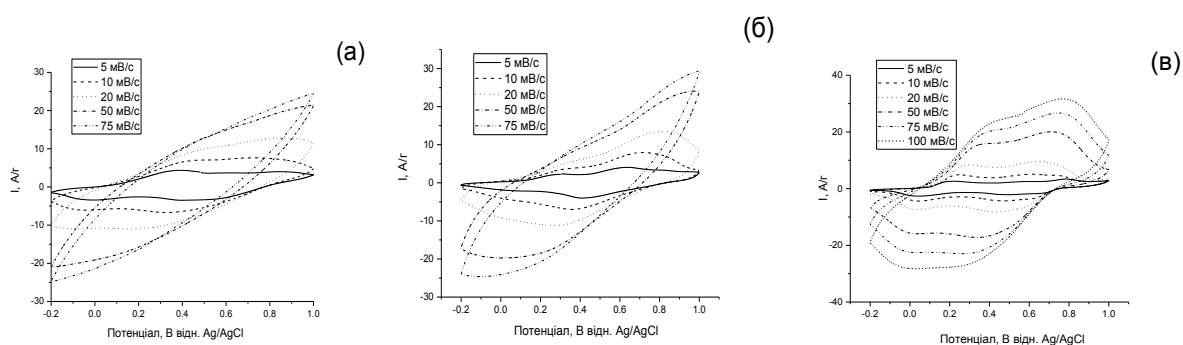
Рис. 6. ЦВА нанокompatитів nMoS_2/ПАН(75) (а), nMoS_2/ПАН(50) (б) і nMoS_2/ПАН(25) (в) при різних швидкостях розгортки потенціалу
