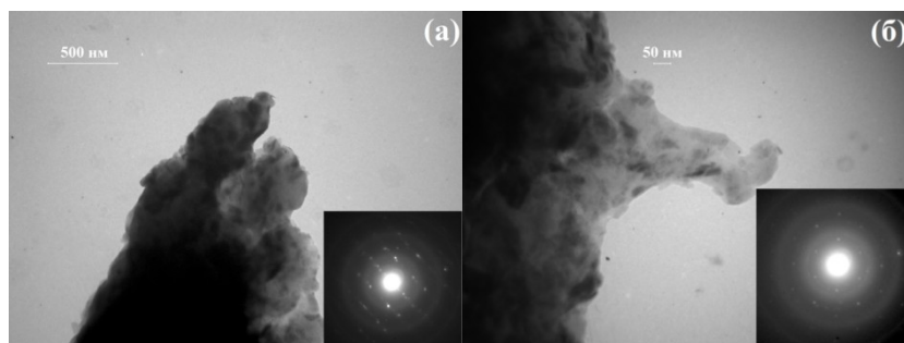
Рис. 2. ТЕМ зображення частинок нанокompatитів n\text{WS}_2/\text{ПАН}(75) (а) та n\text{WS}_2/\text{ПАН}(25) (б)
