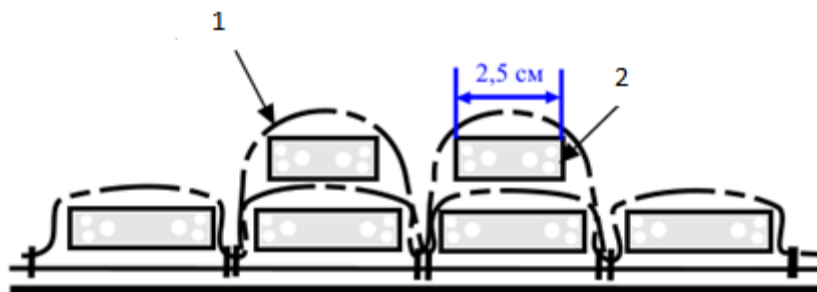
Рис. 2. Схема демпфіруючого шару на другому зразку: 1 – другий шар сітки, 2 – демпфіруючий шар
