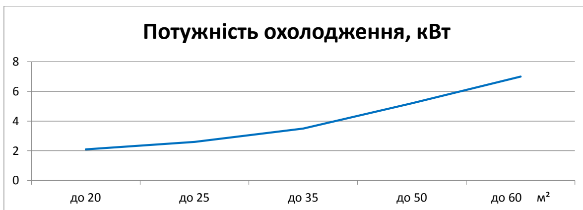
Рис. 3. Графік залежності потужності охолодження від площі приміщення
