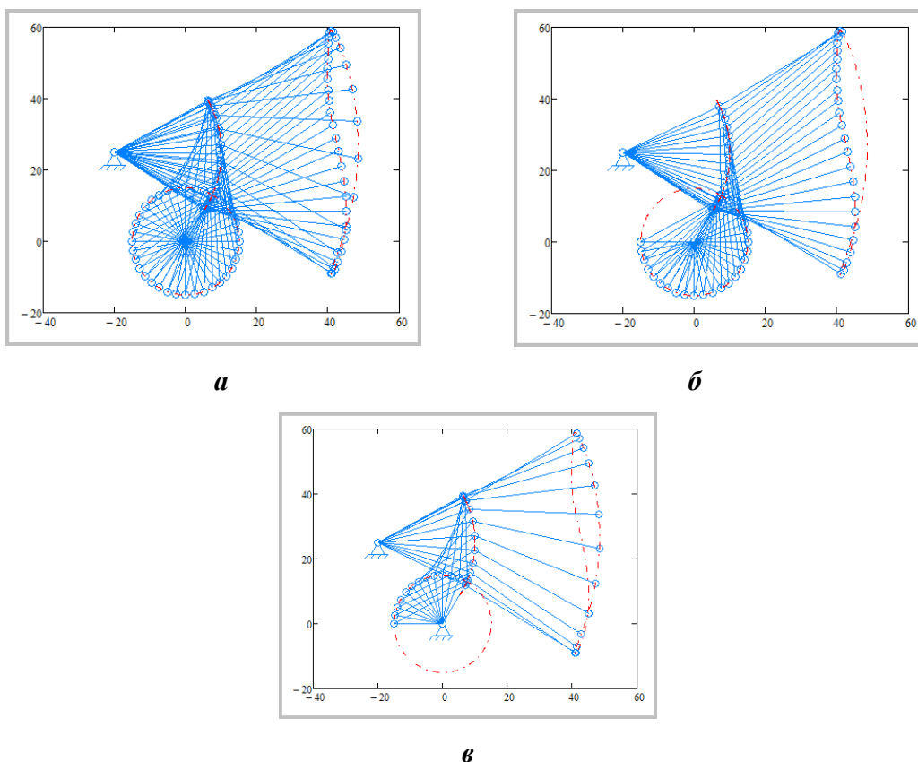
Рис. 3. Візуалізація схематехнічного моделювання механізму ниткопритягача швейної машини для: a – 36 положень; б – 24 положення на фазовому куті подачі нитки; в – 12 положень на фазовому куті виведення нитки
