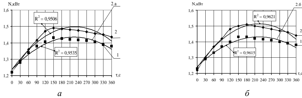
Рис. 2. Энергозатраты при тестоприготовлении: а – влажность теста W 43%; б – влажность теста W 45 %; 1 — месильного органа новой конструкции; 2 – базовый месильный орган; 2.а – 1 аппроксимирующая кривая N = -4 \cdot 10^{-06} \tau^2 + 0,01\tau + 1,24 ; 2.а – 2 аппроксимирующая кривая N = -5 \cdot 10^{-06} \tau^2 + 0,02\tau + 1,24 ; 2.б – 1 аппроксимирующая кривая N = -4 \cdot 10^{-06} \tau^2 + 0,02\tau + 1,24 ; 2.б – 2 аппроксимирующая кривая N = -5 \cdot 10^{-06} \tau^2 + 0,003\tau + 1,24
