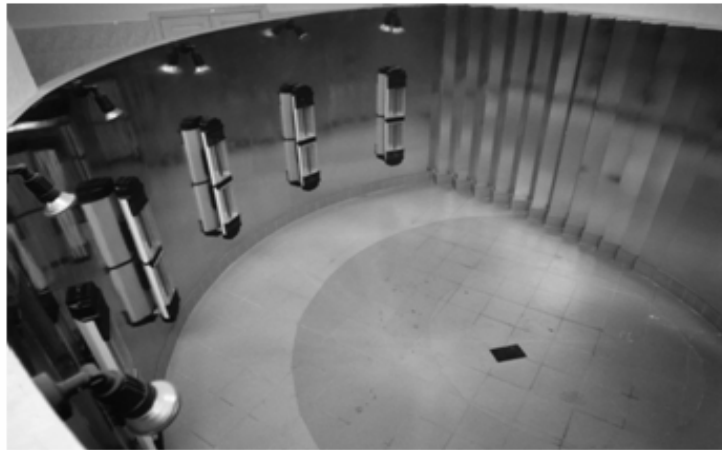
Рис. 5. Камера пелоидотерапии с угловыми и цилиндрическим отражателями
