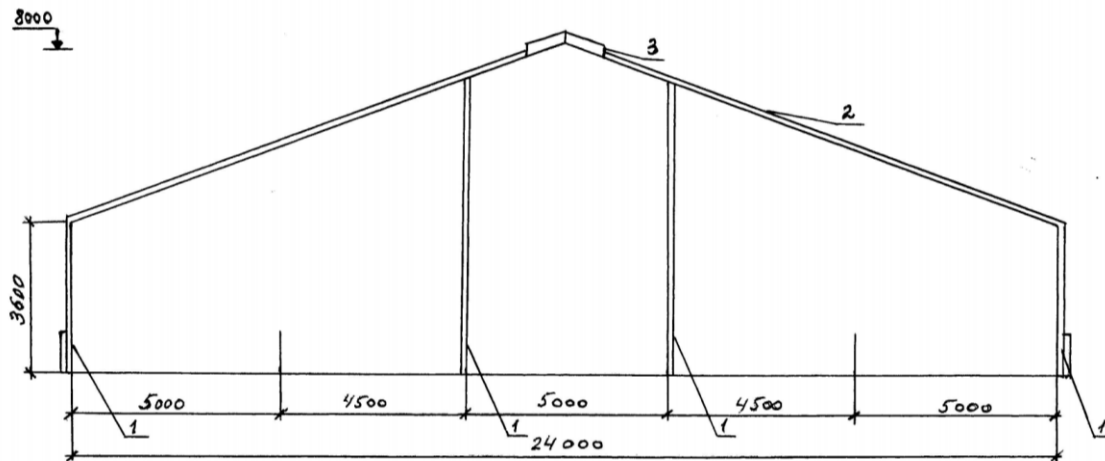
Рис. 1. Поперечний розріз легкозбірної будівлі для відгодівлі молодняка великої рогатої худоби.
