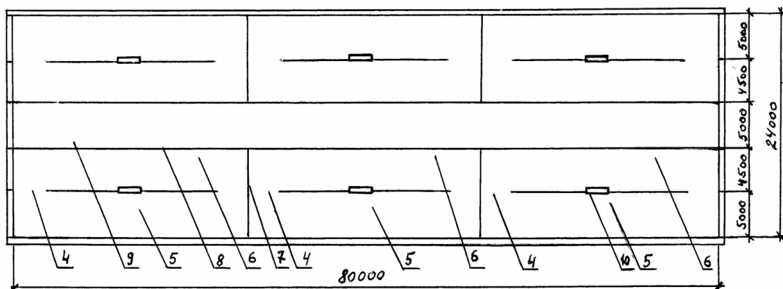
Рис. 2. Секції для утримання відгодівельного молодняка: 1) металеві колони; 2) металеві балки; 3) світло-аераційний дашок; 4) секції для утримання відгодівельного молодняка; 5) зона для відпочинку тварин
