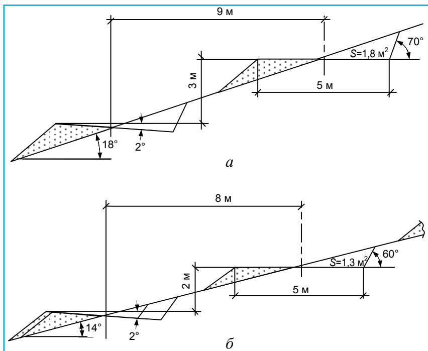
Рис. 1. Схеми терасування відкосів: а – розрізної траншеї; б – відвалів.
