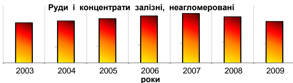
Рис. 2. Динаміка видобутку та вироблення залізородної сировини за 2003–2009 рр., млн т 1
