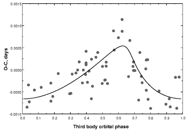
Рис. 3. Кривая блеска в Bessel R-фильтре и график (O-C)
