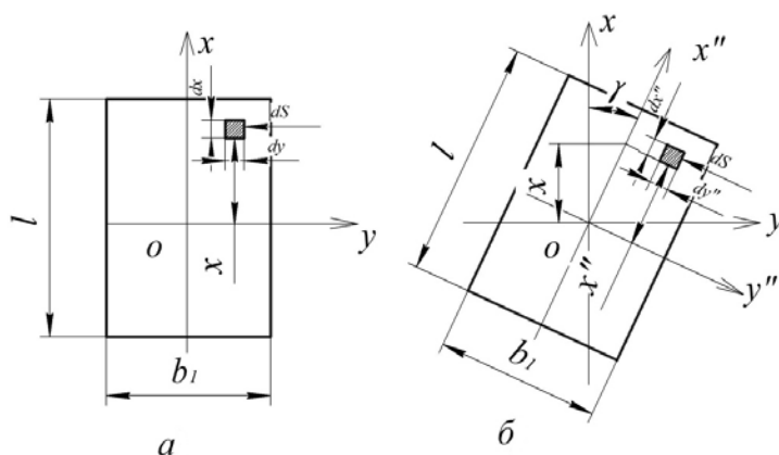
Рисунок 1 – Модель контактной силы, создающей момент сопротивления поворота: a – для неповоротного ведущего колеса; б – для управляемого ведомого колеса.
