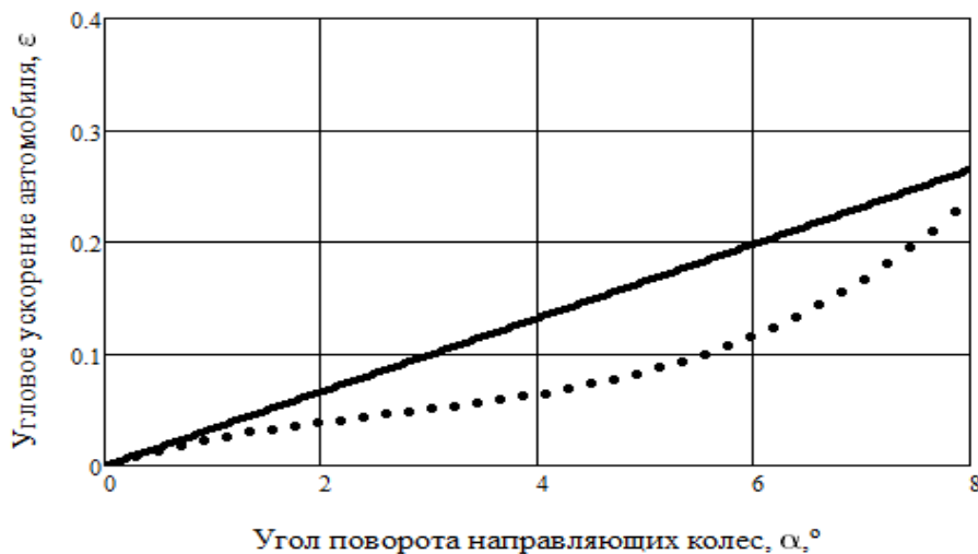
Рисунок 4 – Зависимость углового ускорения автомобиля в плоскости дороги от угла поворота направляющих колес: ••••• с учетом M_{cm} и M_{uu} ; — без учета M_{cm} и M_{uu}
