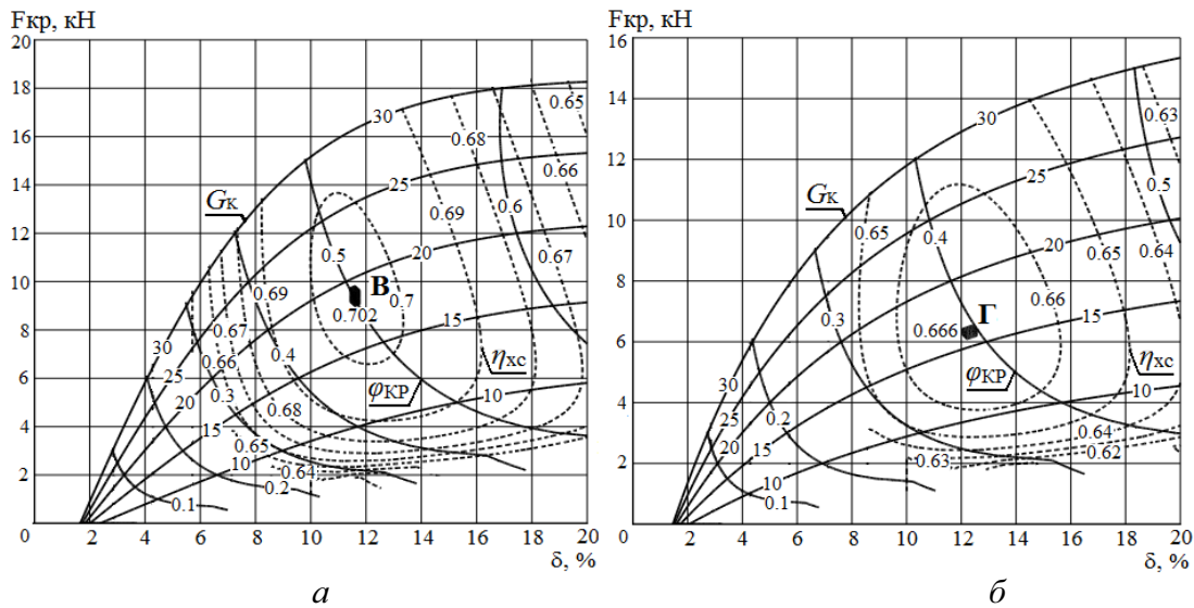
Рисунок 2 – Универсальная характеристика шины 21,3 R24 при давлении в воздухе в шине 0,1 МПа: а – методика [3]; б – методика [4].
