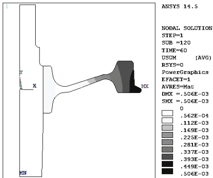
Рисунок 23 – Суммарные перемещения при t = 60 с.
