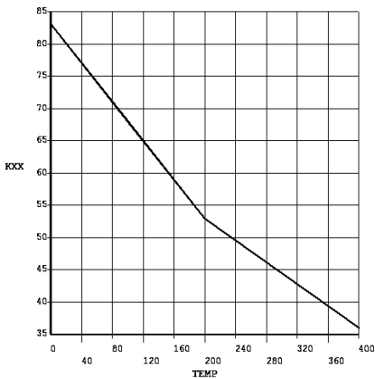
Рисунок 5 – Теплопроводность
