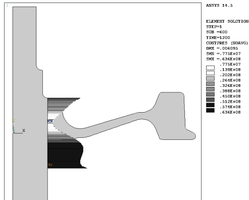
Рисунок 22 – Контактное давление при t = 1200 с.
