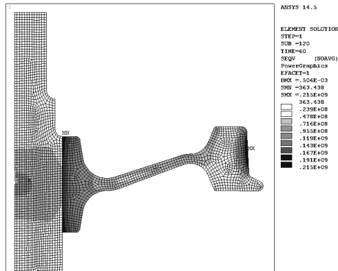
Рисунок 27 – Эквивалентные напряжения при t = 60 с.
