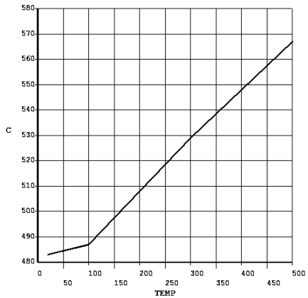
Рисунок 4 – Удельная теплоемкость
