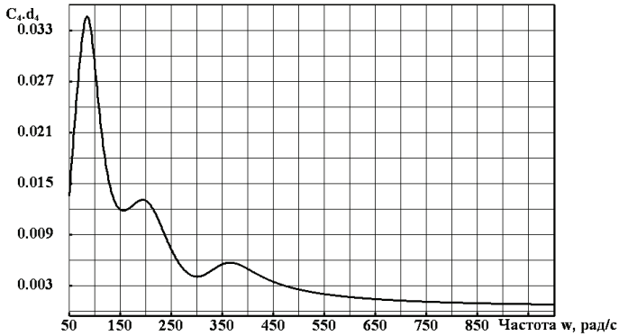
Рисунок 6 – АЧХ 4-го пружного(гідроб'ємний зв'язок) елемента ГСМП
