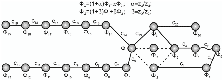
Рисунок 1 – розрахункова схема системи турбонадува двигуна
