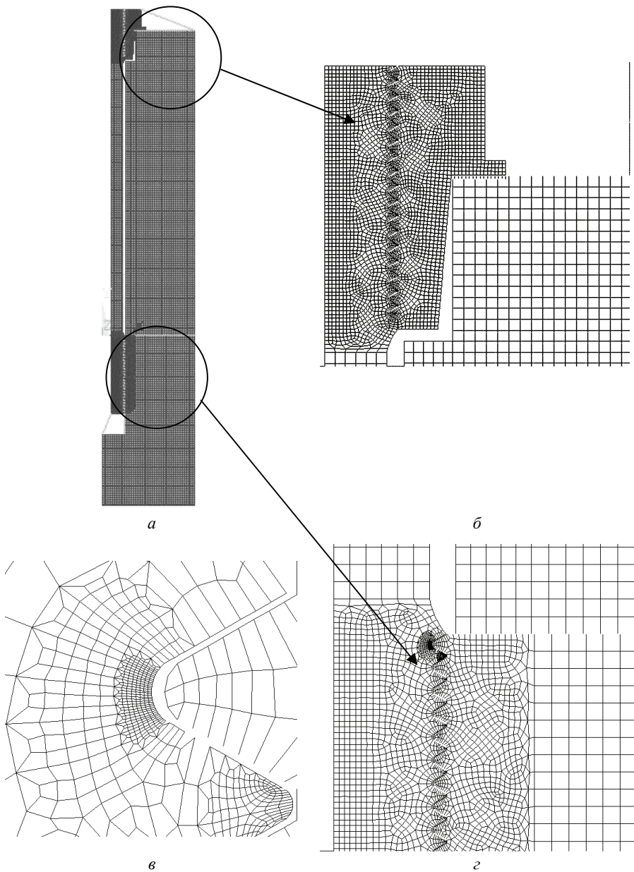
Рисунок 3 – Скінчено-елементна осесиметрична модель шпилькового з'єднання:
