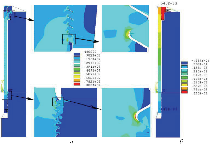
Рисунок 5 – Напруження та переміщення для осесиметричної моделі шпильки: a – напруження по Мізесу, Па, б – переміщення, м
