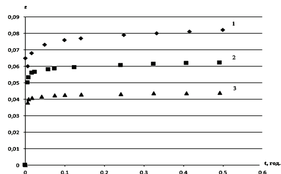
Рисунок 3 – Залежність повної деформації зразку від часу. Зразки, що вирізано вздовж напрямку прокатки
