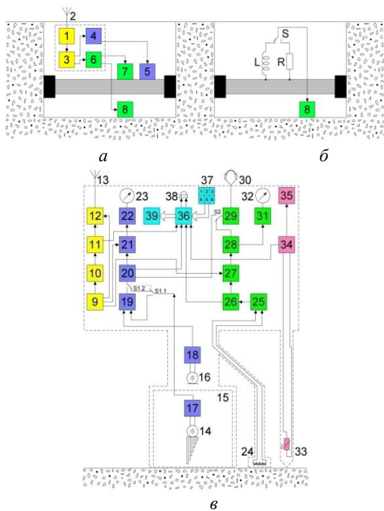
Рис. 1 – Функціональна схема ІВС: a – вузол збудження; б – вузол навантаження; в – вимірювальний вузол
