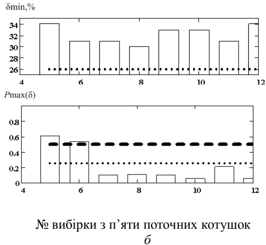
Рис.2 – Результати контролю відносного видовження при розриві \delta : a – мінімальне значення \delta_{min} , визначене для п'яти поточних котушок і обмежене знизу: \delta_{min} > 26\% (пунктир); б – контрольна карта максимальної ймовірності виходу параметра за нормативну границю P_{max}(\delta)
