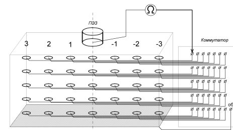
Рис. 4 –Схема раскладки датчиков и измерительной цепи
