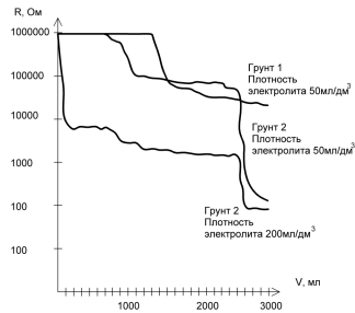
Рис. 5.– Совмещённый график изменения сопротивления для цепи "заземлитель – подстилающая пластина" при различном типе грунта и концентрации электролита
