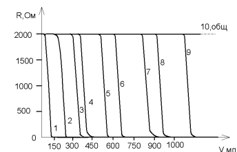
Рис. 2 – Зависимость изменения сопротивления «ПЭЗ – датчик (сетка)» от объёма влитого электролита: 1-10 общ - номера сеток
