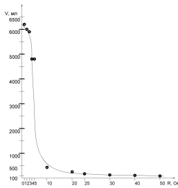
Рис. 8 – Зависимость сопротивления заземлителя от объёма влитого электролита
