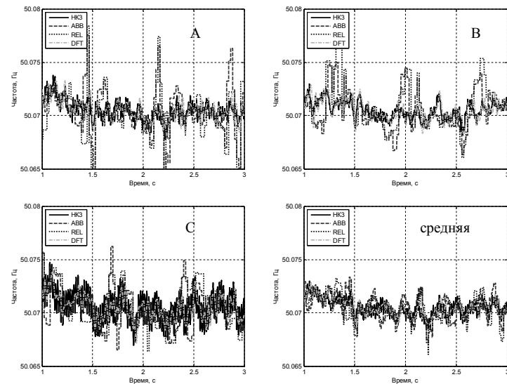
Рис. 2 – Результаты измерения частоты в фазах А, В, С и среднее значение
