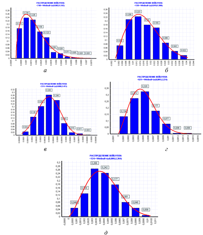
Рис. 4 – Гістограми емпіричного розподілу й функції щільності розподілу Вейбулла для однорідних підмножин газів, розчинених у маслі бездефектних трансформаторів: а – зміст метану; б – зміст етилену; в – зміст етану; г – зміст ацетилену; д – зміст водню.
