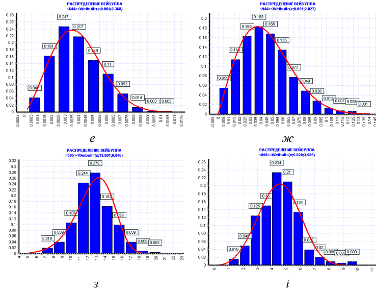
Рис. 5 – Гістограми емпіричного розподілу й функції щільності розподілу Вейбулла для однорідних підмножин газів, розчинених у маслі бездефектних трансформаторів: е – зміст оксиду вуглецю; ж – зміст діоксиду вуглецю; з – зміст азоту; і – зміст кисню.
