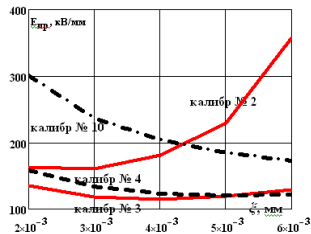
Рис. 5 – Расчетные зависимости максимальной напряженности электрического поля от размера дефекта для различных экспериментально определенных значений толщины изоляции
